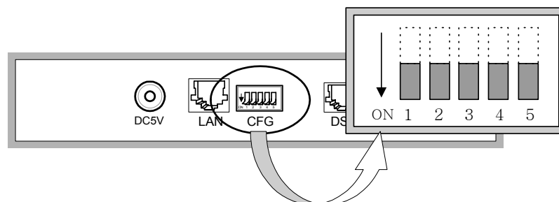
Фабричные настройки DIP-переключателей.
